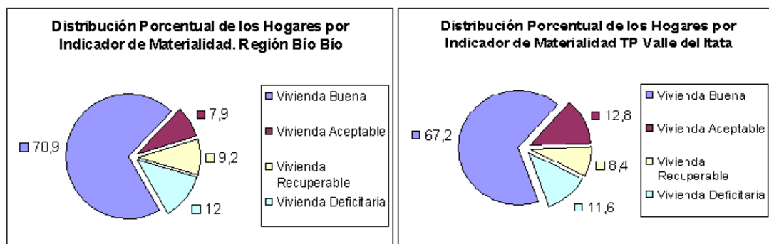
Ilustración 15: Gráfico comparado del Indicador de Materialidad Regional y TPVI 8
